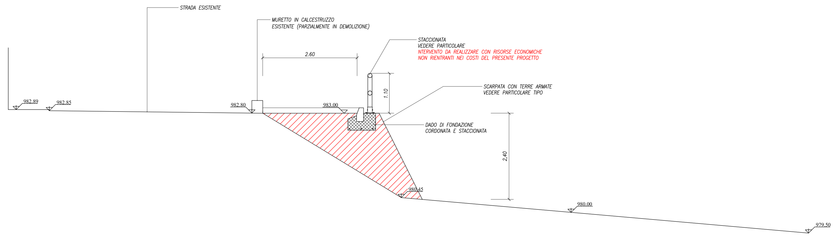
SEZIONE SC. 1:50
